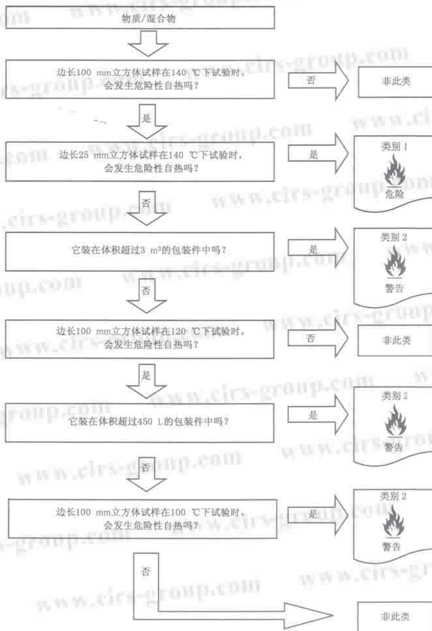
图 A.1 自热物质和混合物判定逻辑
